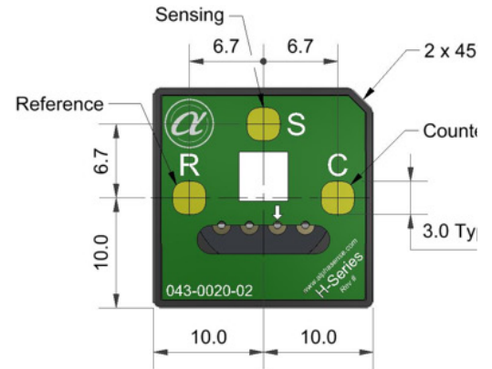
底视图
